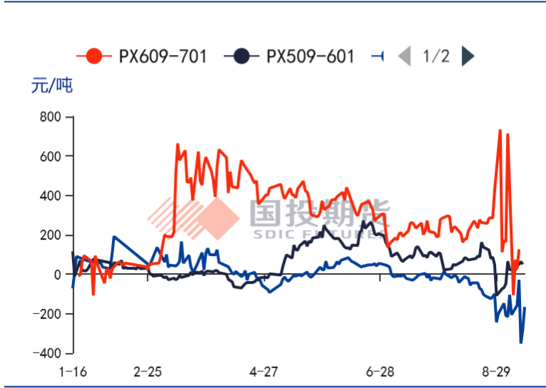
图6：PX9-1月差
