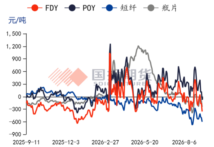
图16：聚酯利润
