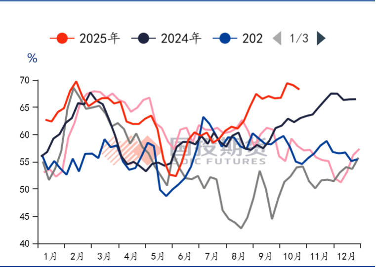
图27：隆众乙二醇周度开工率
