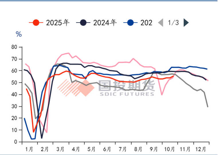
图31：国内纺织开工率
