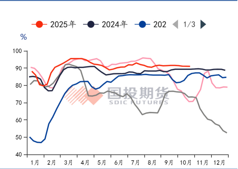
图29：隆众长丝开工率
