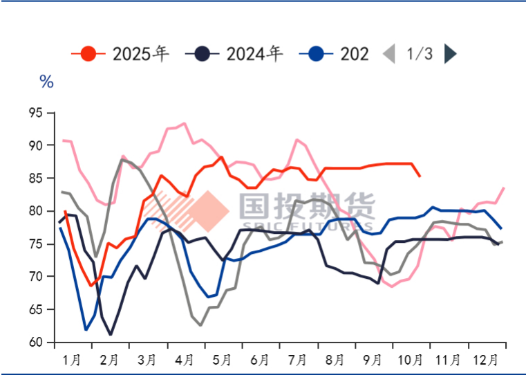
图28：隆众短纤开工率
