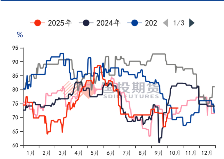
图30：PET瓶片日度开工率
