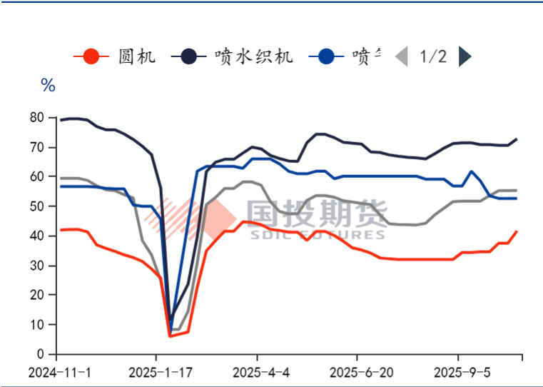
图32：下游织造开工率
