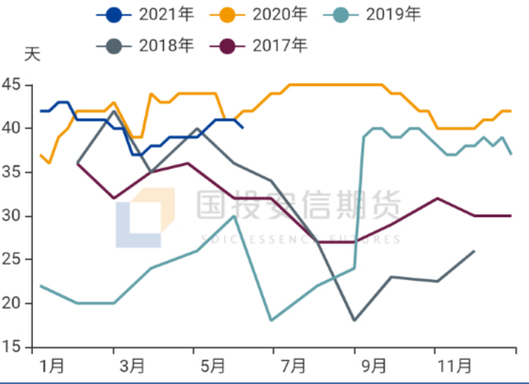
图32：华东坯布周度库存
