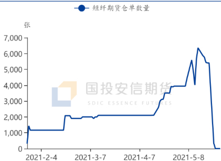
图29: 短纤期货仓单数量
